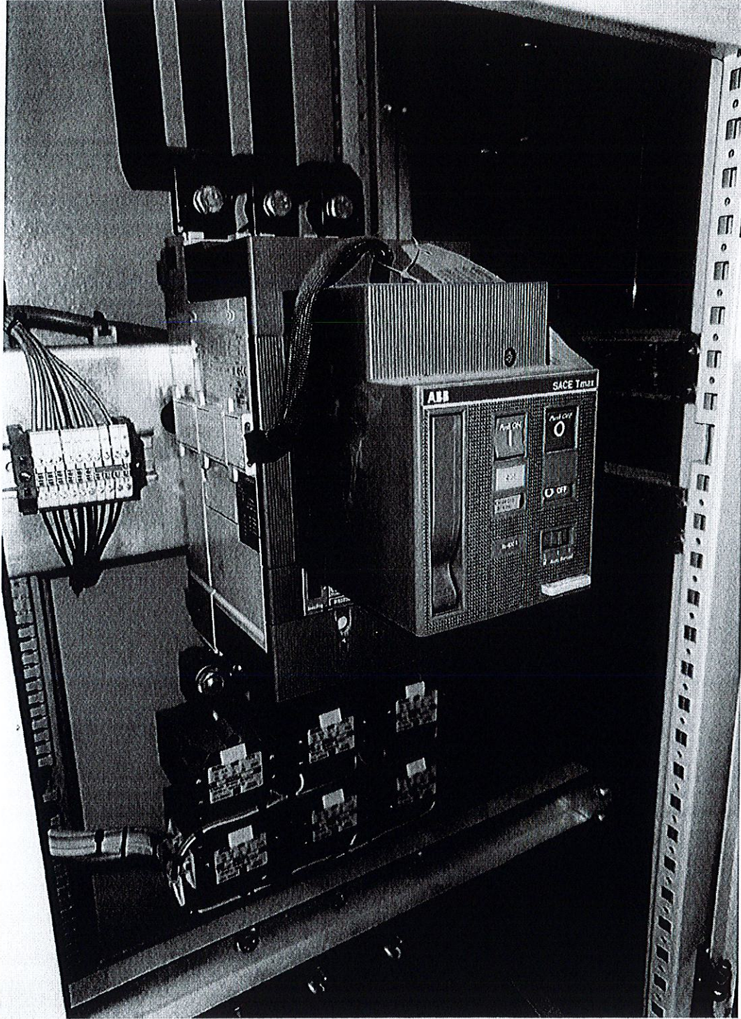
Resim 6 Mevcut Şalter - Bara Bağlantı Düzeni
