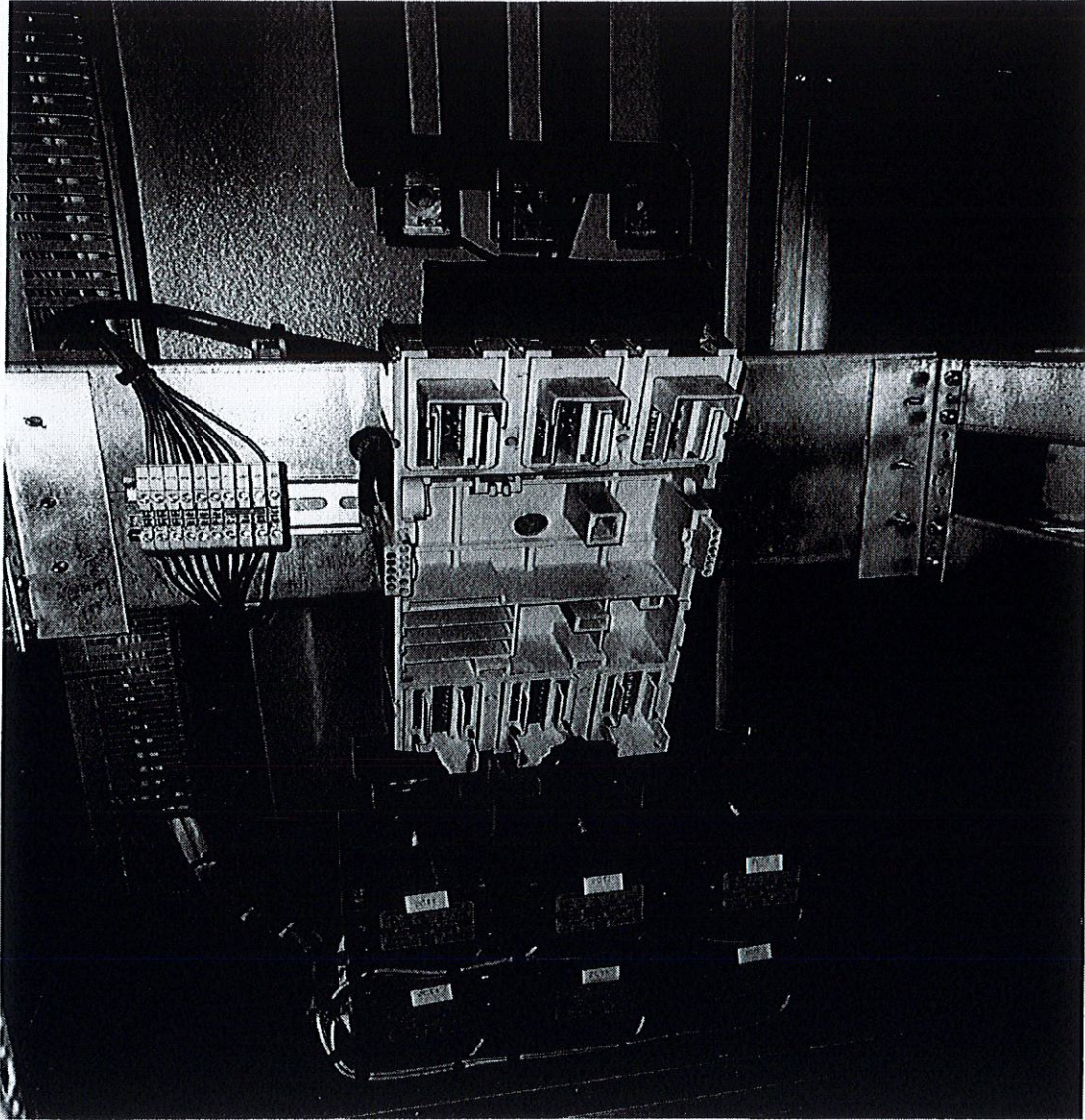
Resim 1 Mevcut Şalter Bağlantı Kasası
