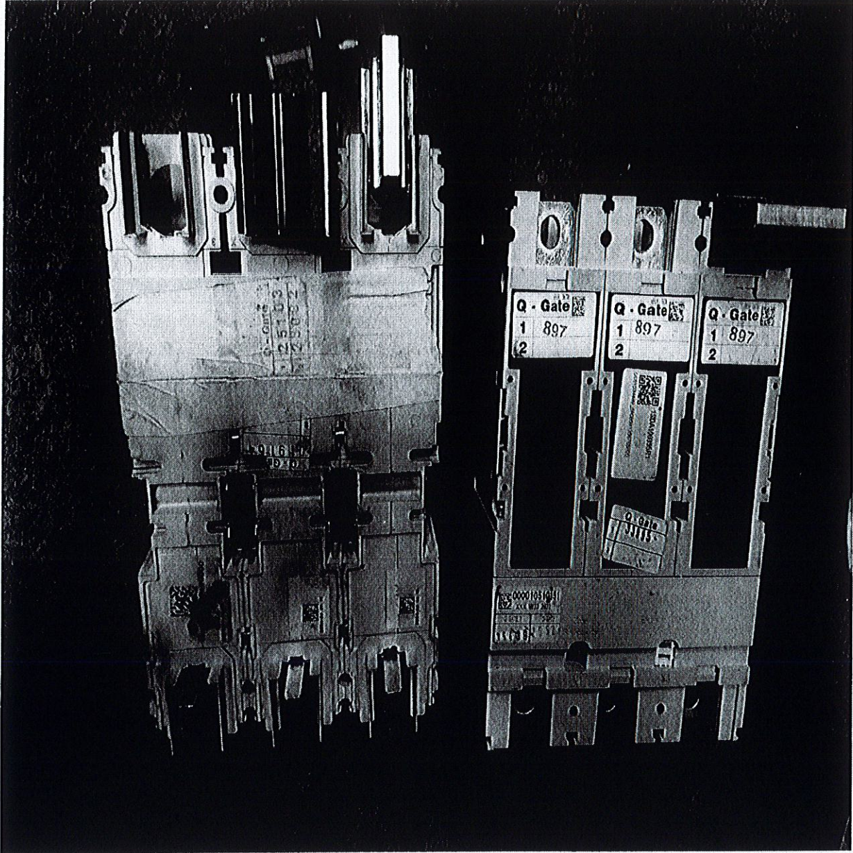
Resim 5 Soldaki eski arızalı şalter, sağdaki yeni kullanılacak şalter ve eski şaltere uygun pimler
