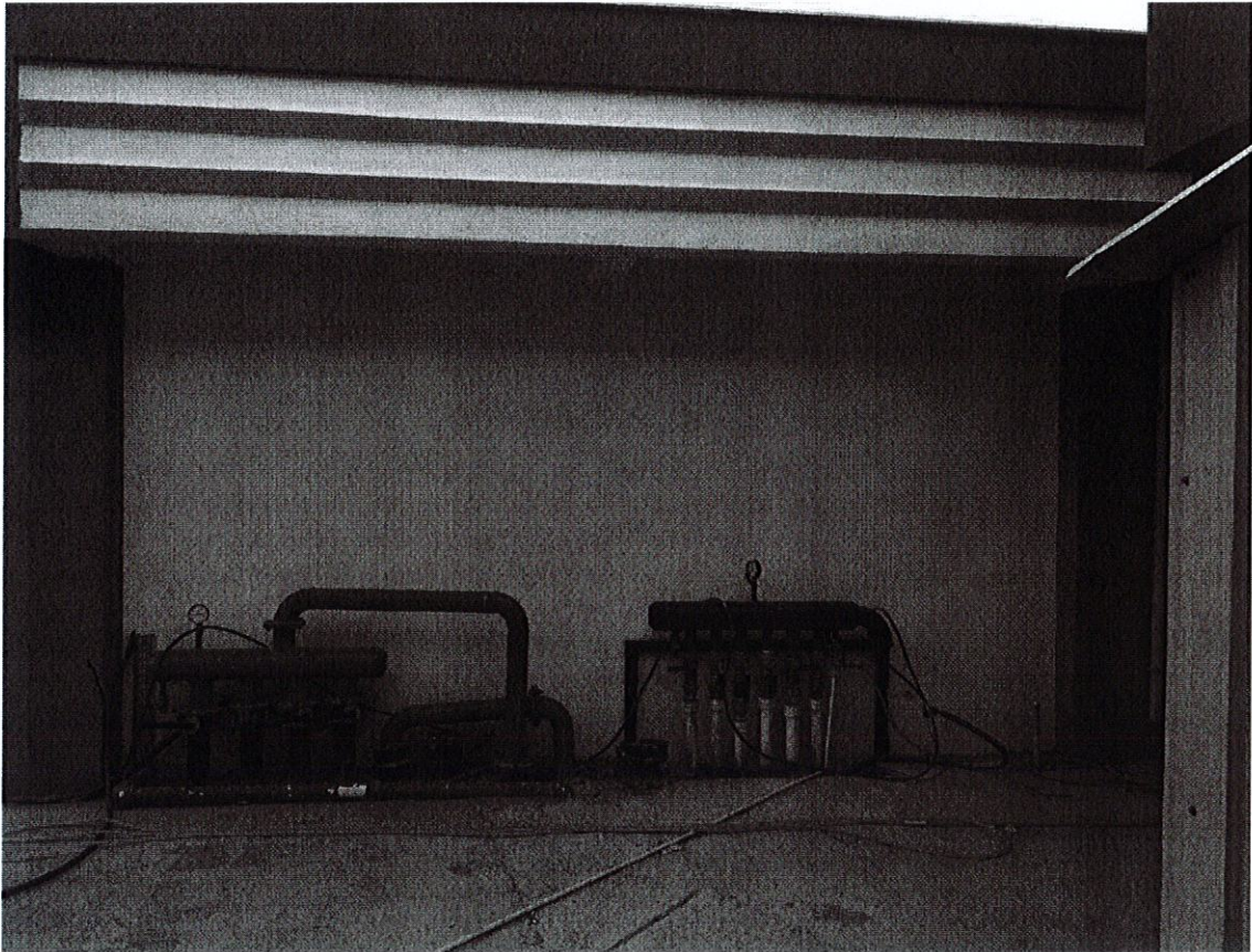
Yangın istasyonu valf ve boru devreleri, kolektör kısmı görünümü
