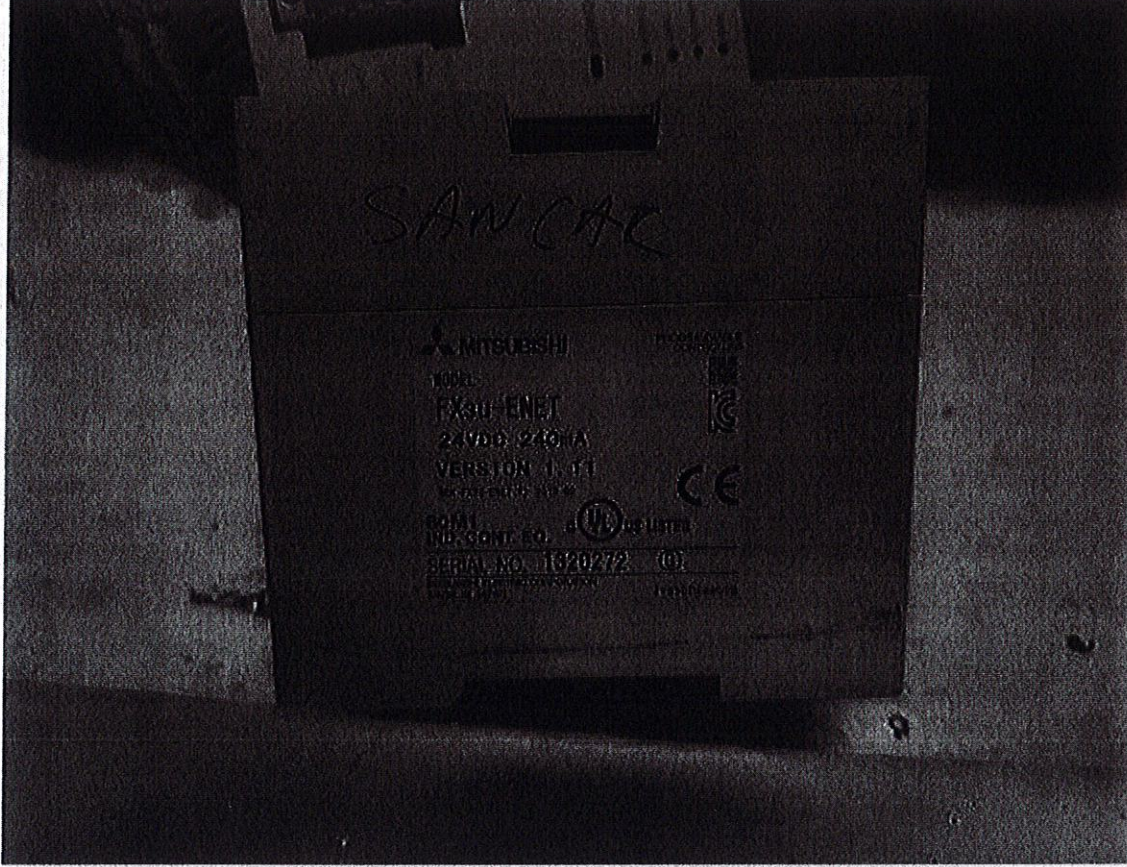
MODÜL 3.ÜNİTE-Mitsubishi- Model: FX 3U-ENET-24 VDC 240 mA (ETHERNET INTERFACE)
